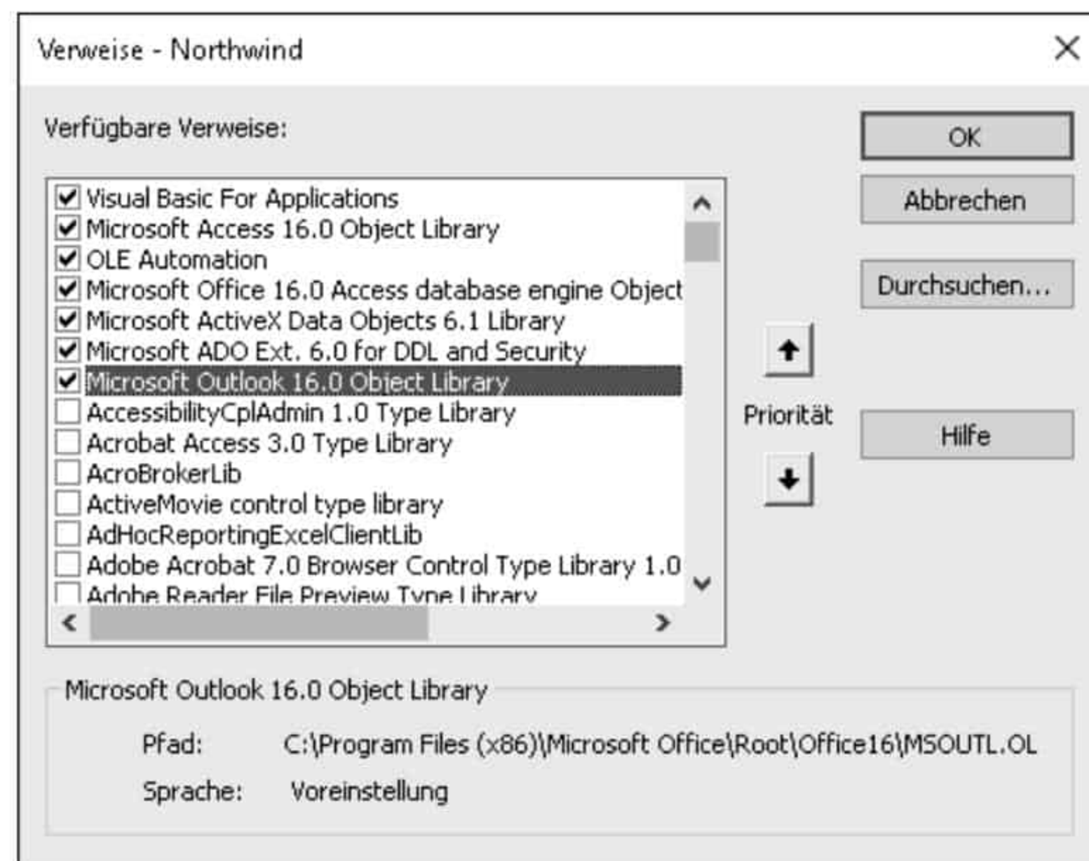
Abbildung 10.25 Die Outlook-Bibliothek einbinden
