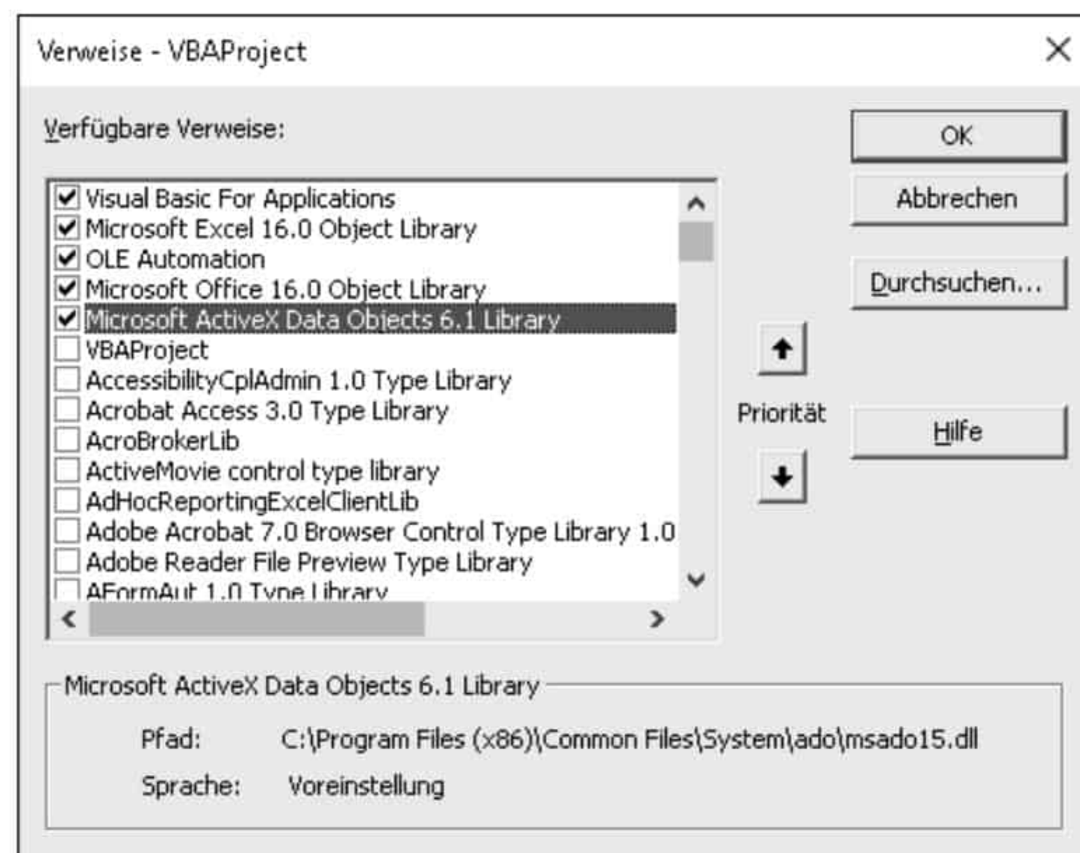
Abbildung 10.40 Die ADO-Bibliothek einbinden
