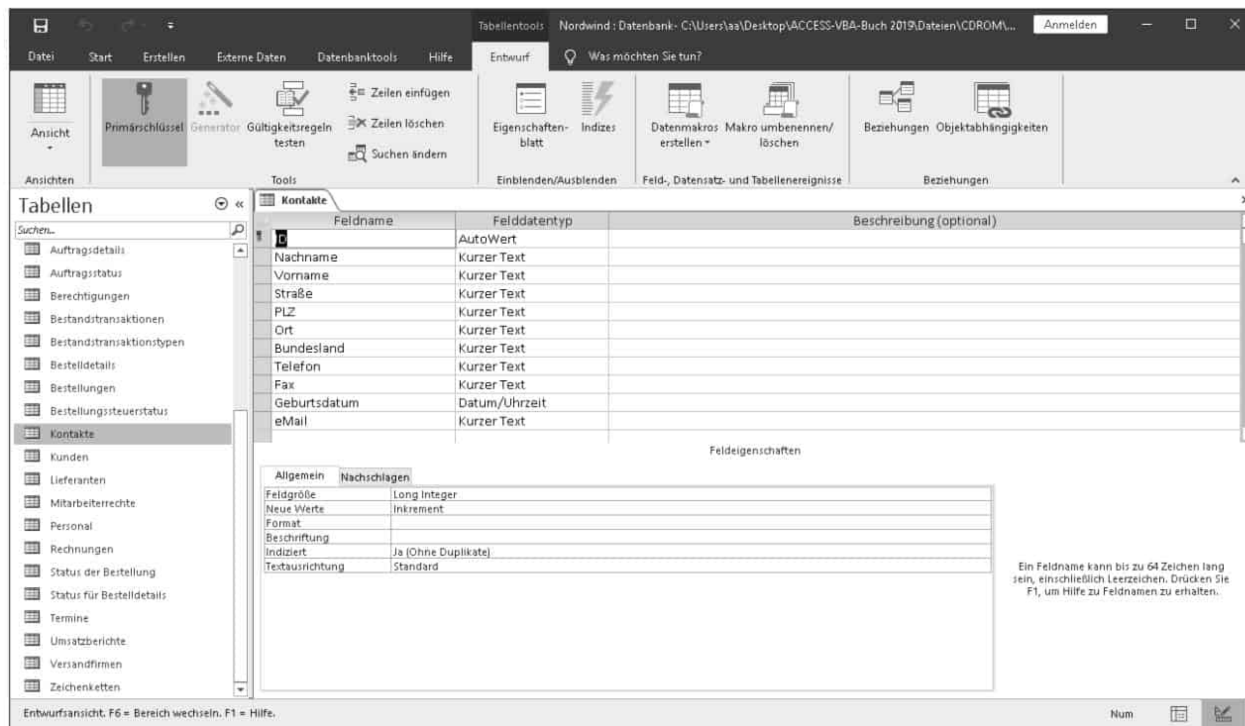
Abbildung 10.23 Der Aufbau der Adressentabelle in der Entwurfsansicht
