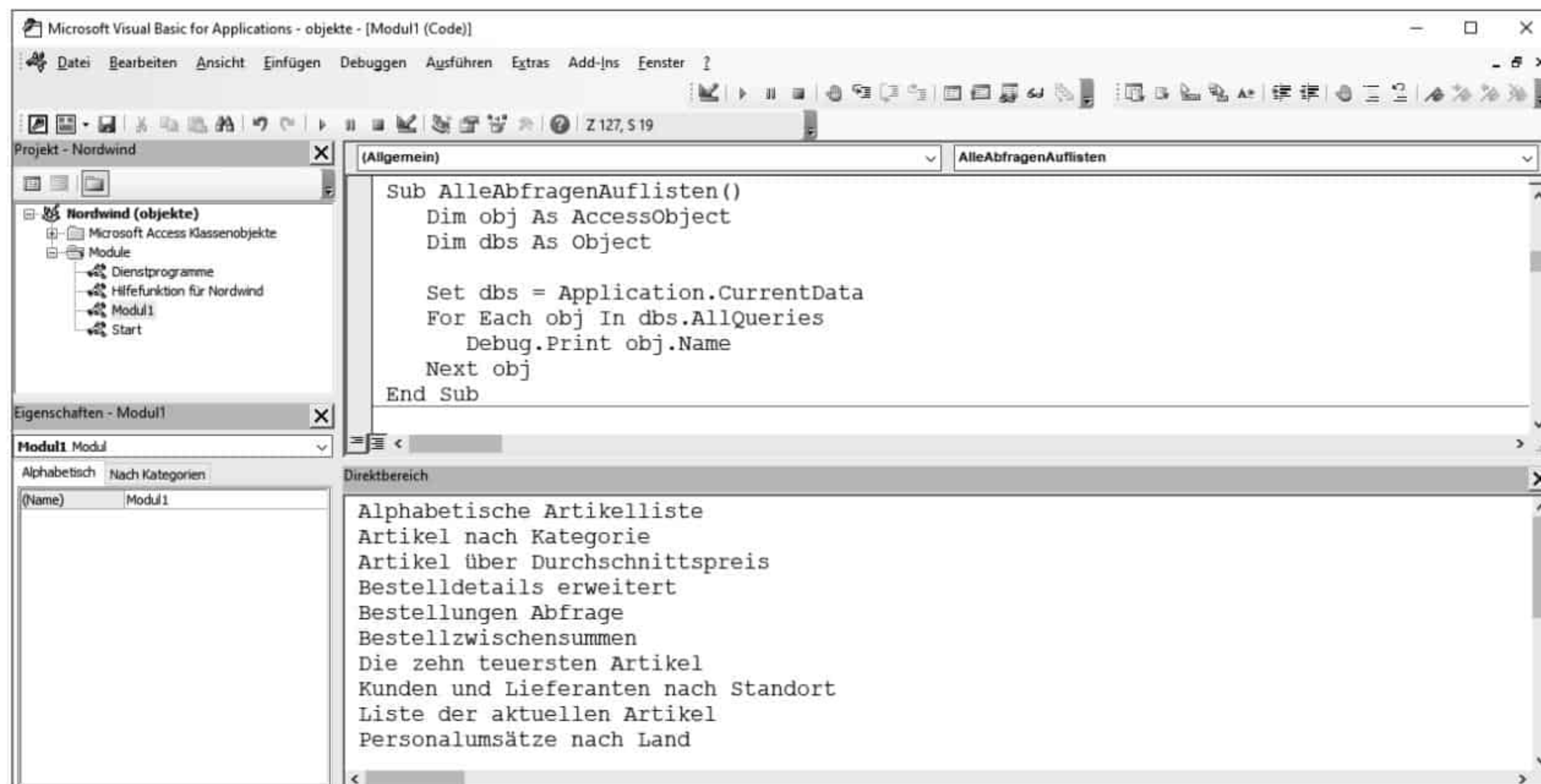
Abbildung 4.6 Den Namen, das Erstellungs- sowie das Änderungsdatum der geöffneten Tabellen herausfinden
