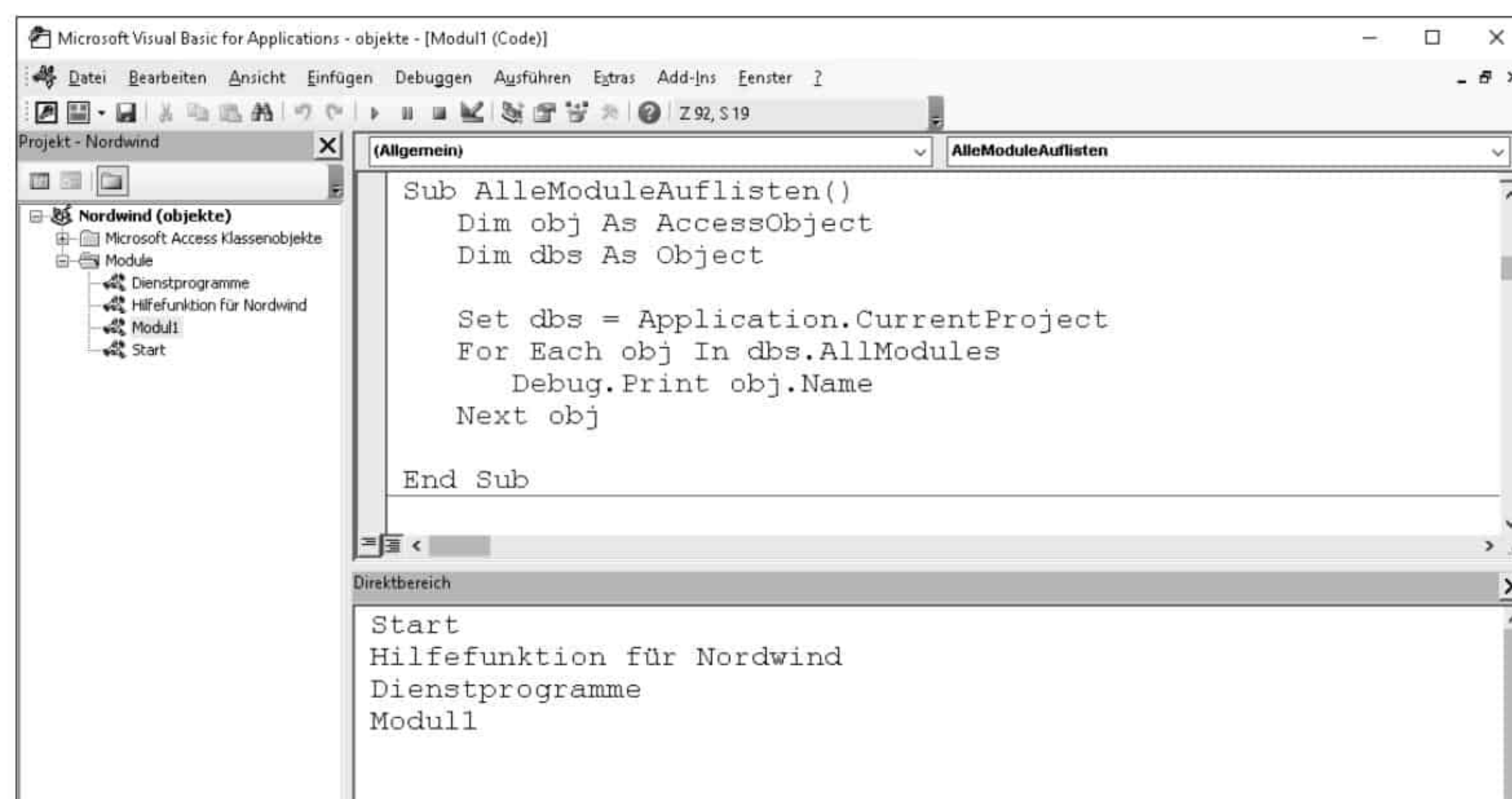
Abbildung 4.5 Alle Module der Datenbank im Direktfenster ausgeben
