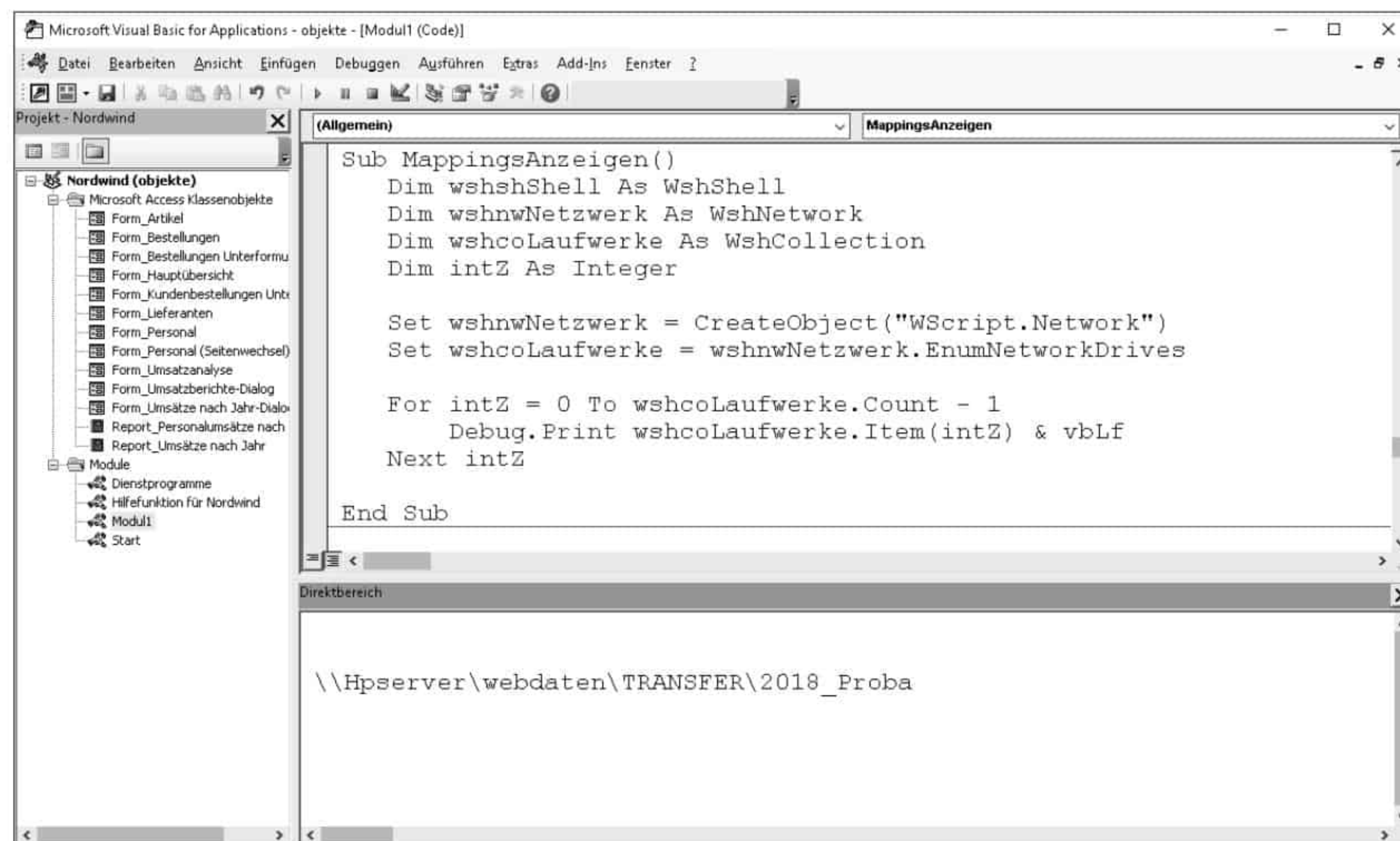
Abbildung 4.17 Alle Mappings anzeigen
