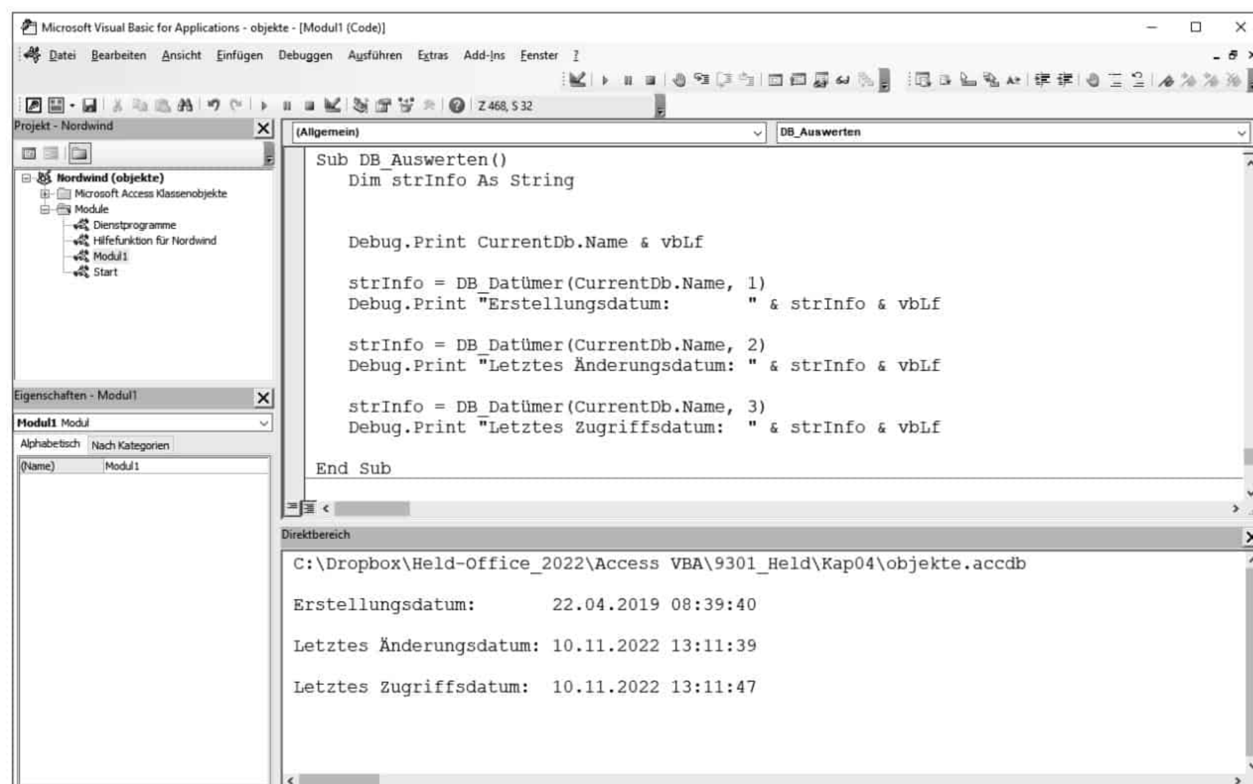
Abbildung 4.20 Alle Informationen zur aktuellen Datenbank
