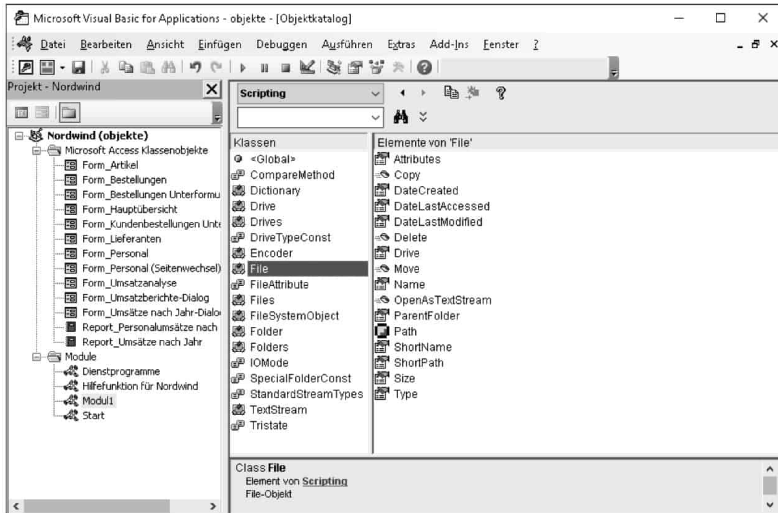
Abbildung 4.14 Alle Methoden und Eigenschaften für die Dateibearbeitung
