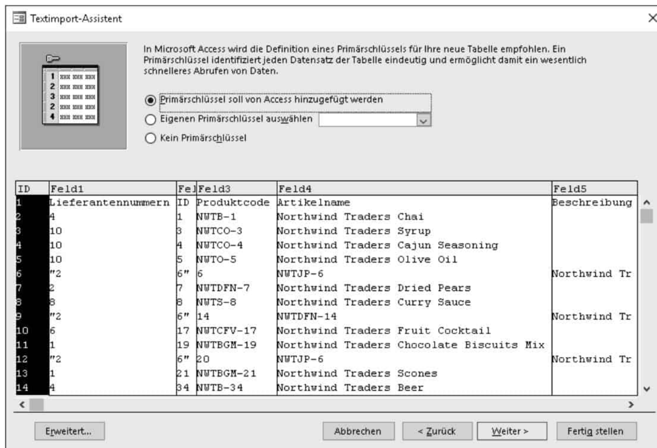
Abbildung 10.13 Ein Primärschlüssel kann angelegt werden.
